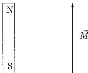
Figura 1: Um ímã em barra e seu momento de dipolo magnético
