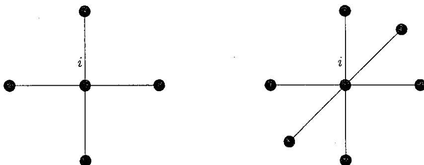
Figura 5: Número de primeiros vizinhos em d = 2 e d = 3
