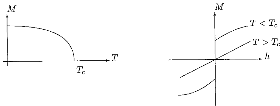
Figura 2: Comportamento da magnetização M com a temperatura T e com o campo magnético externo h
